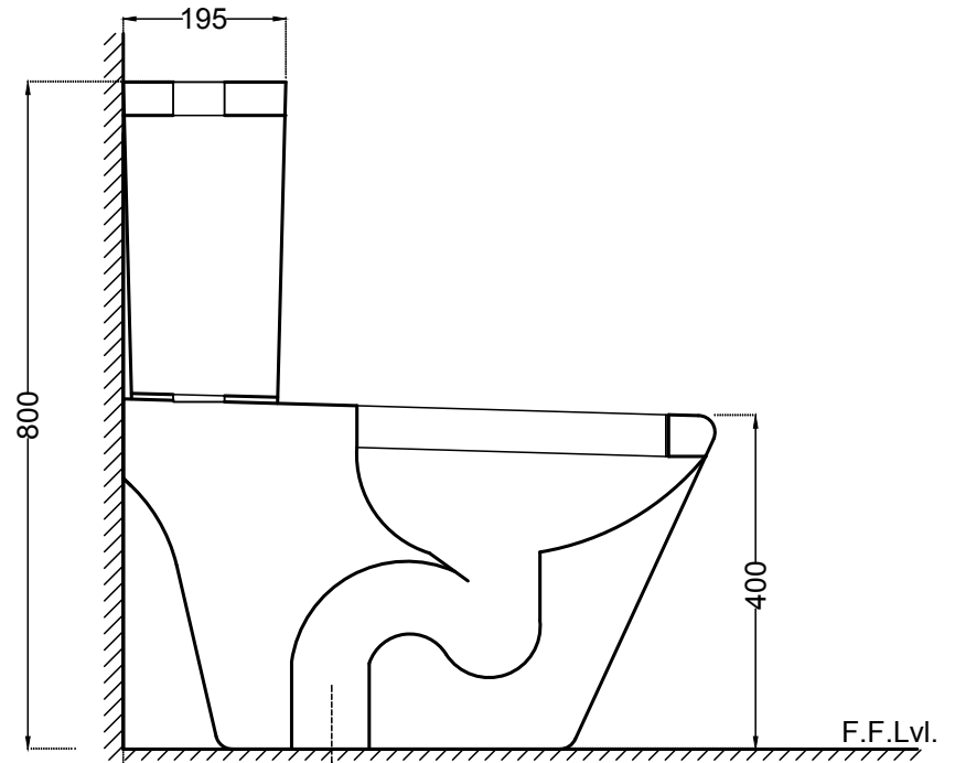
S TRAP - 250
